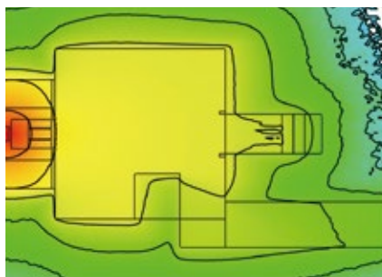
図2 左端ターゲット付近から広がる線量分布(遮蔽計算)
