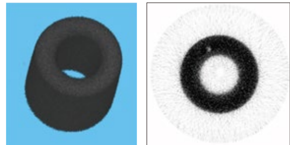
図2 直径1mmの穴をあけた銅のシリンダーの中性子CT再構成結果と断面図
