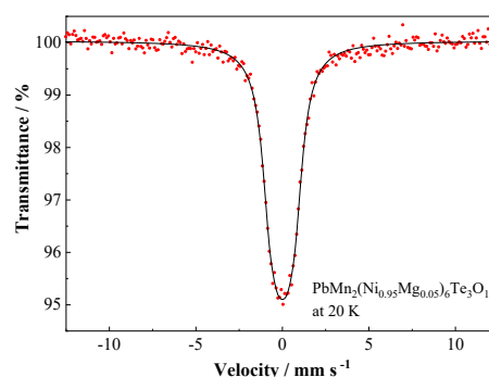
Fig. 1. The ^{61}\text{Ni} Mössbauer spectrum of Mg-doped \text{PbMn}_2\text{Ni}_6\text{Te}_3\text{O}_{18} .
