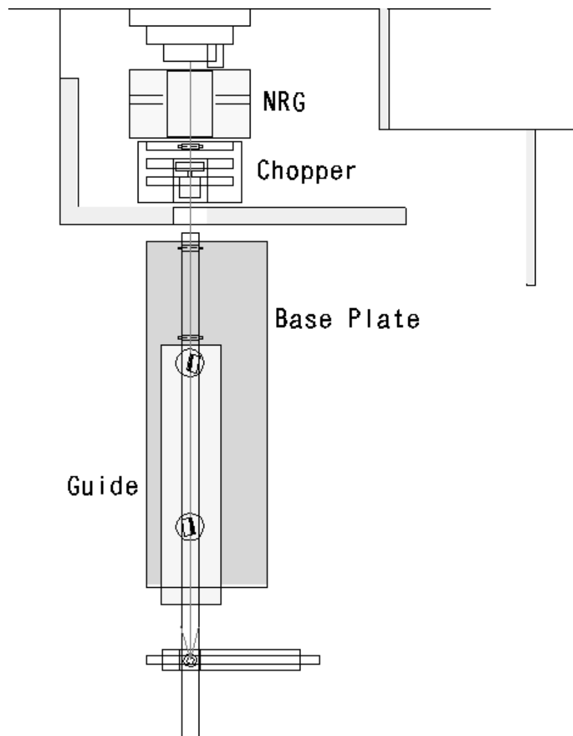
第 4 図 C N - 3 実験孔における飛行時間法利用モード配置
