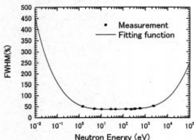
図4 KULSのエネルギー分解能
