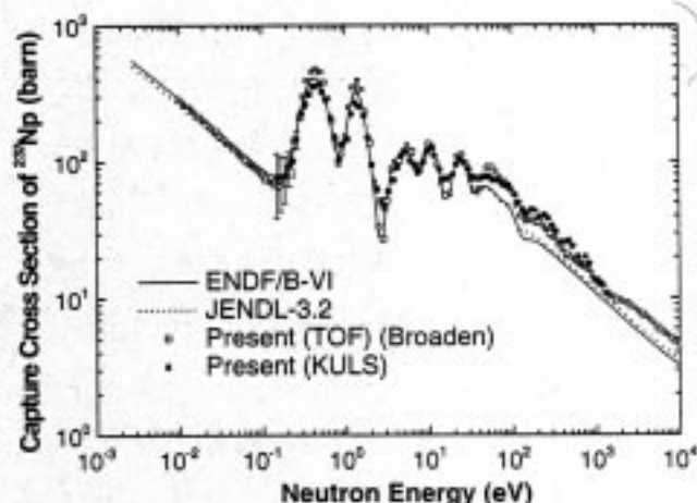
図9 ^{237}\text{Np}(n,\gamma) 反応断面積
