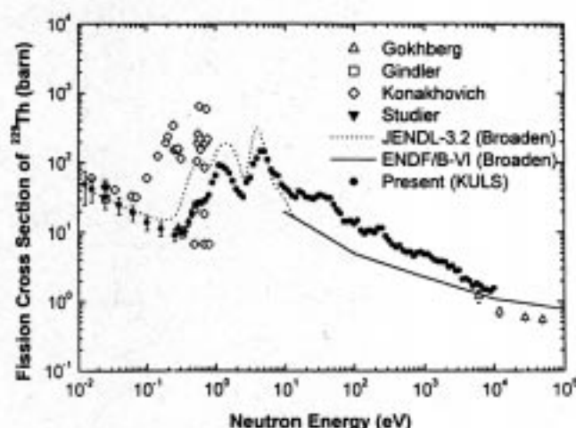
図7 ^{229}\text{Th}(n,f) 反応断面積
